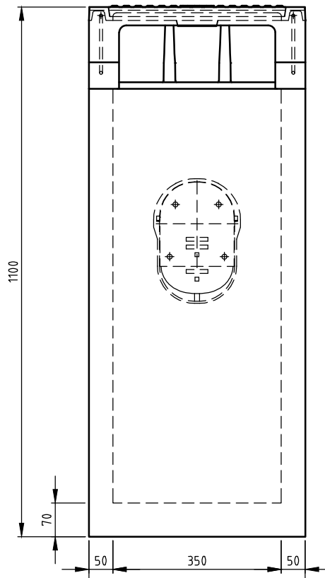
VOORAANZICHT
