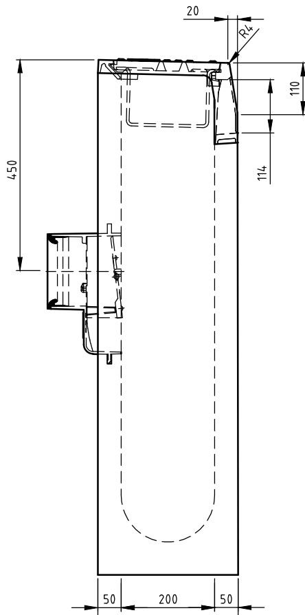
ZIJ-AANZICHT
