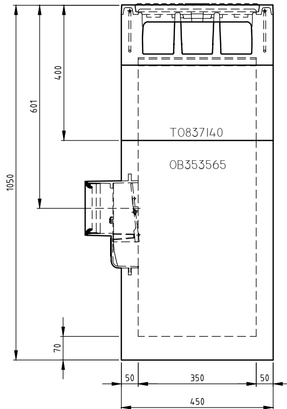
VOORAANZICHT
