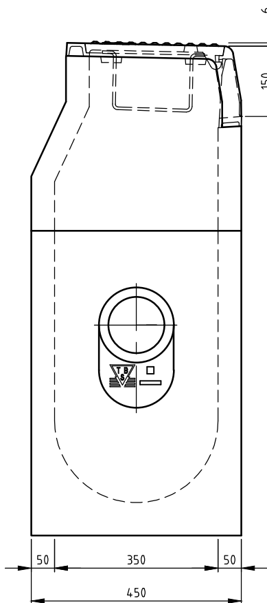
ZIJ-AANZICHT
