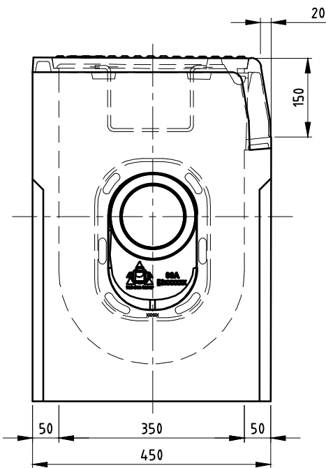
ZIJEAANZICHT
