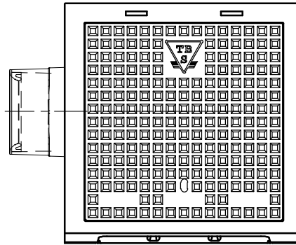
BOVENAANZICHT
