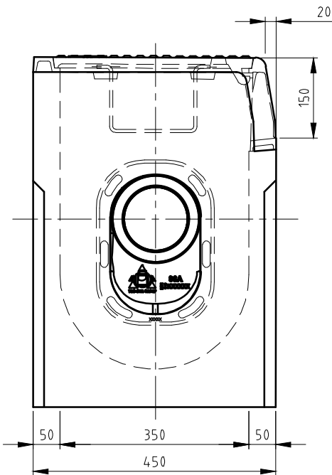
ZIJAANZICHT
