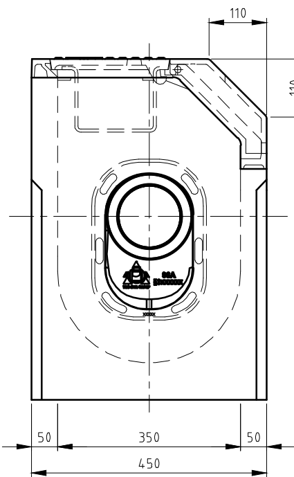
ZIJEAANZICHT
