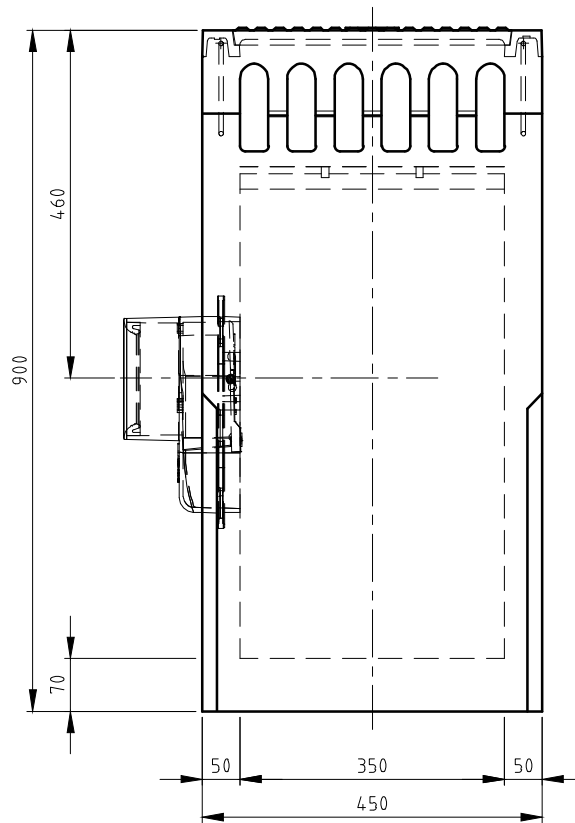
VOORAANZICHT
