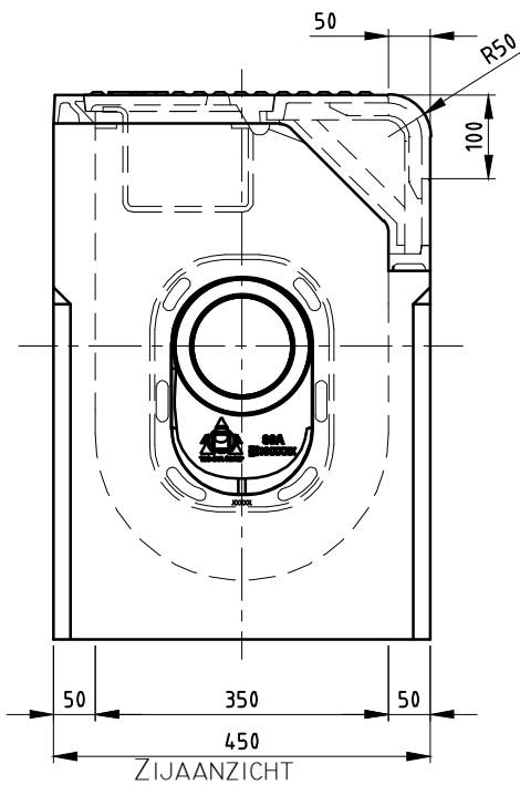
ZIJEAANZICHT
