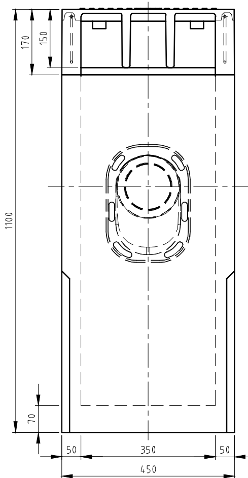
VOORAANZICHT
