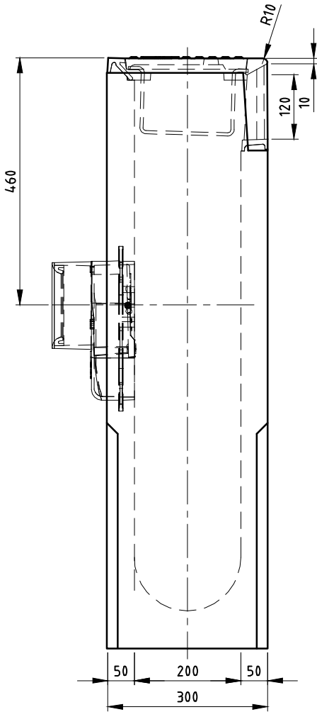
ZIJAAANZICHT
