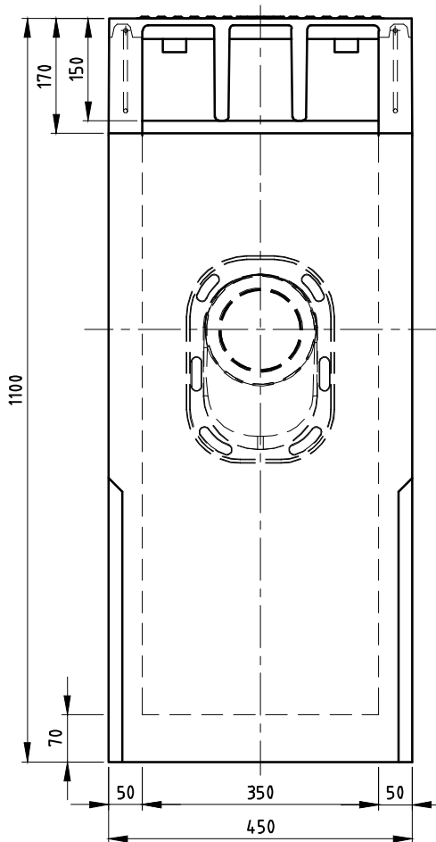
VOORAANZICHT
