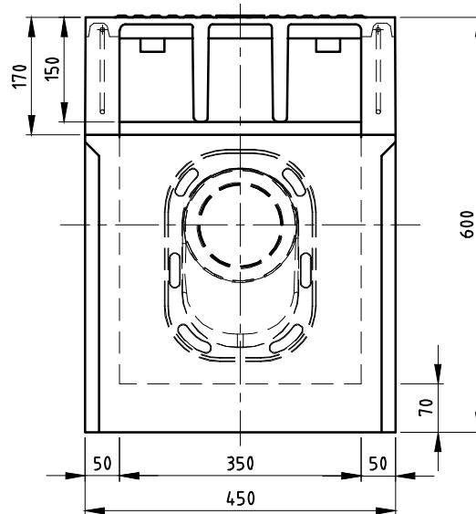
VOORAANZICHT
