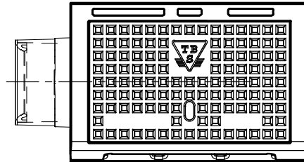
BOVENAANZICHT
