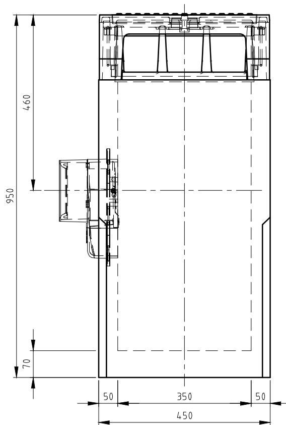
VOORAANZICHT
