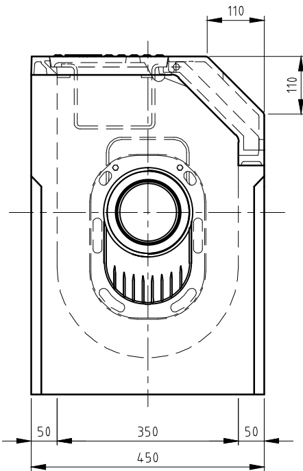
ZIJEAANZICHT
