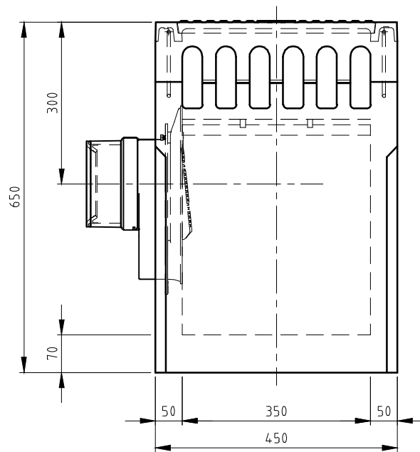
VOORAANZICHT
