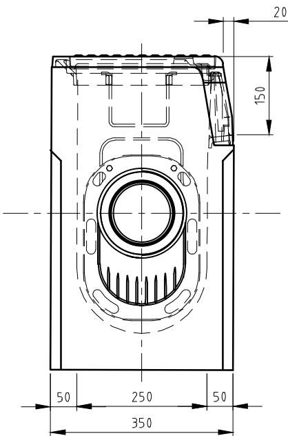
ZIJAAANZICHT
