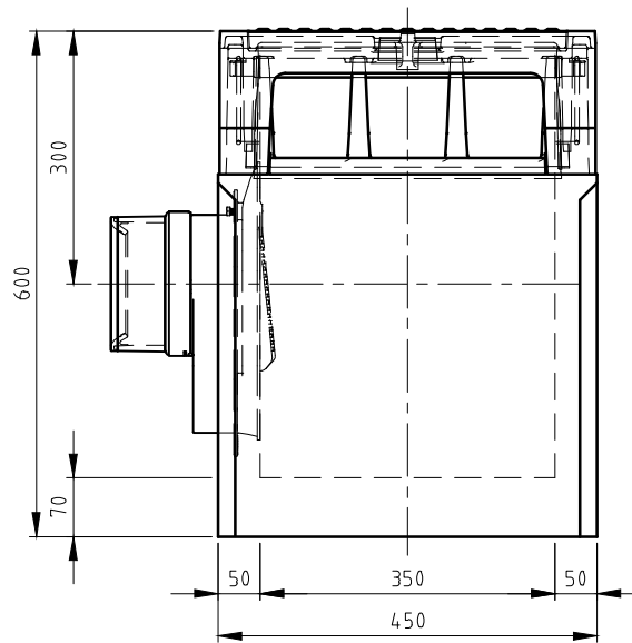
VOORAANZICHT
