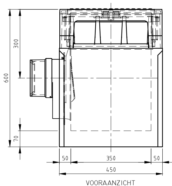
VOORAANZICHT
