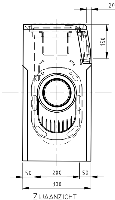
ZIJAAANZICHT
