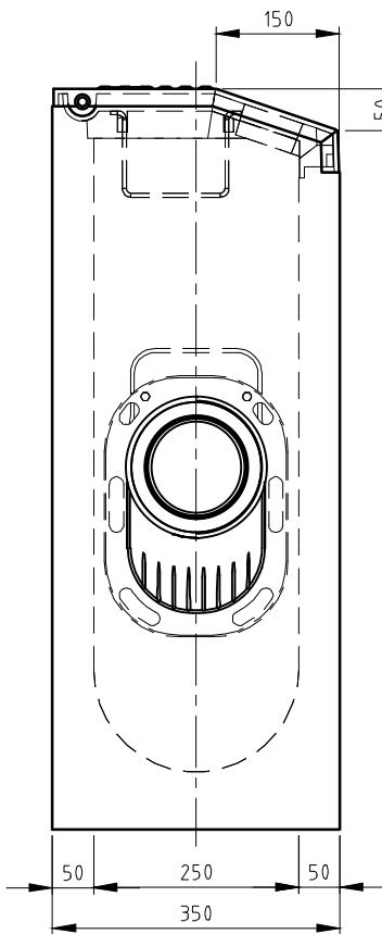
ZIJAANZICHT
