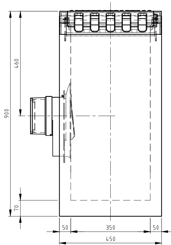
VOORAANZICHT
