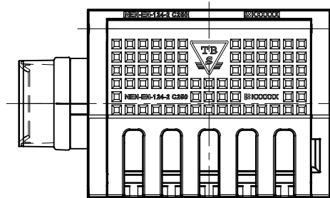
BOVENAANZICHT
